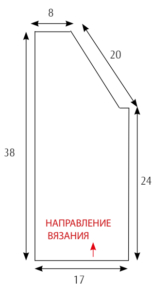
ПЕРЕД
