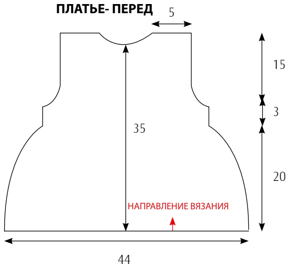
ПЛАТЬЕ - ПЕРЕД
