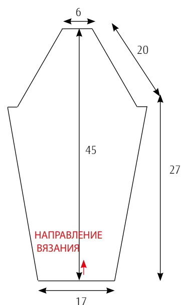
РУКАВ
